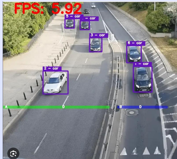
Yolo
