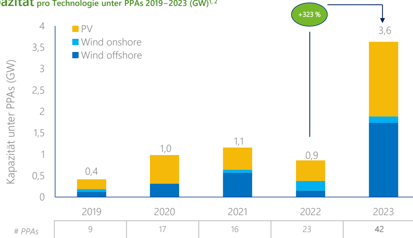
Kapazität pro Technologie unter PPAs 2019–2023 (GW) 1, 2
