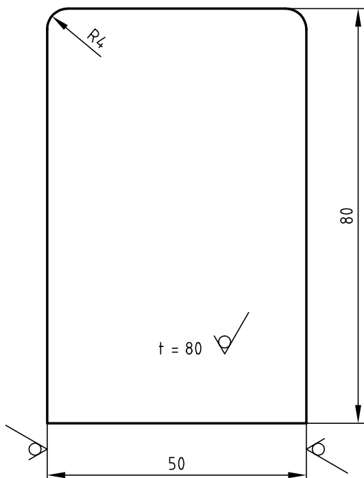
Zeichnung 3 Biegeklotz
